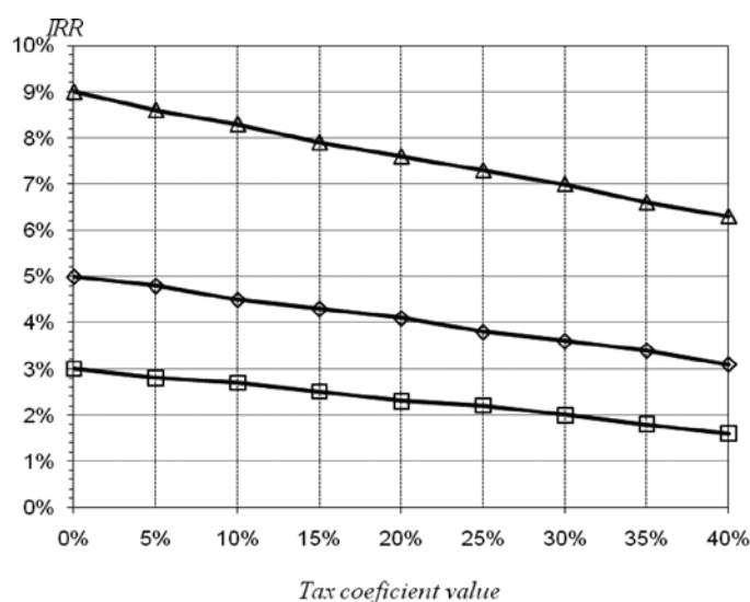
Figura 5.4 - Tasso IRR (%) come funzione dei valori dei coefficienti di tassazione percentuali per i casi A (linea più in alto), B (linea intermedia) e C (linea più in basso).
