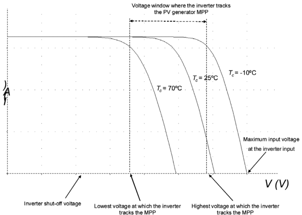
Fig. 3.1. - Curve tensione – corrente di un generatore PV a diverse temperature delle celle ( T_c ), stessa irradianza ( G ), insieme alle tensioni caratteristiche dell'inverter. N.B. : nella figura è stata trascurata l'influenza di secondo ordine che la temperatura della cella esercita sulla corrente di corto circuito.
