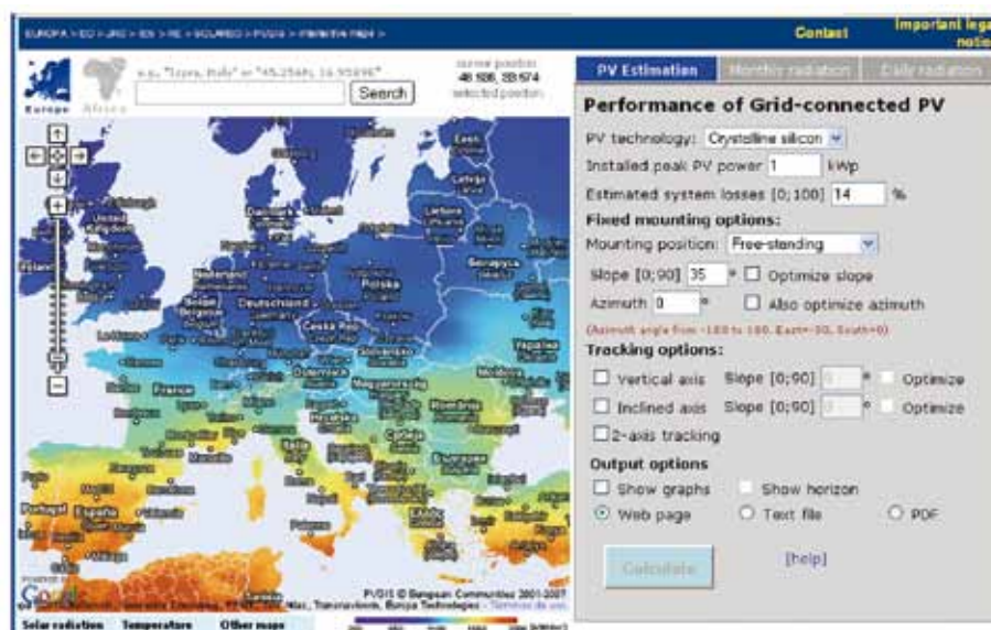
Figura 2.5 - Applicazione web per stimare l'irradiazione inclusa nel sito web PVGIS. (Fonte: http://re.jrc.ec.europa.eu/pvgis/apps3/pvest.php# ).
